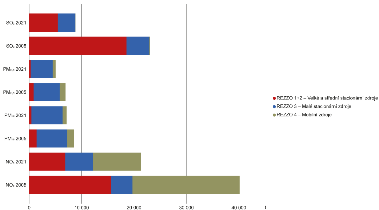
Porovnání zdrojů emisí [t], 2005 a 2021
