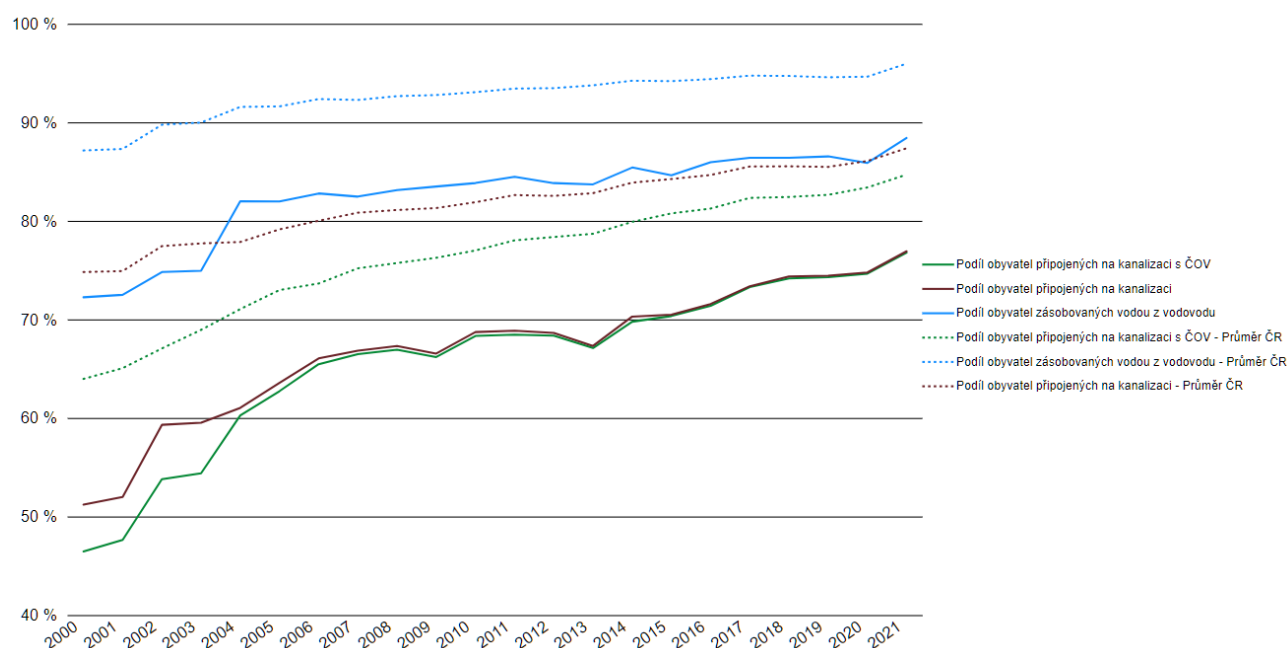
Podíl obyvatel připojených na vodohospodářskou infrastrukturu [%], 2000–2021
