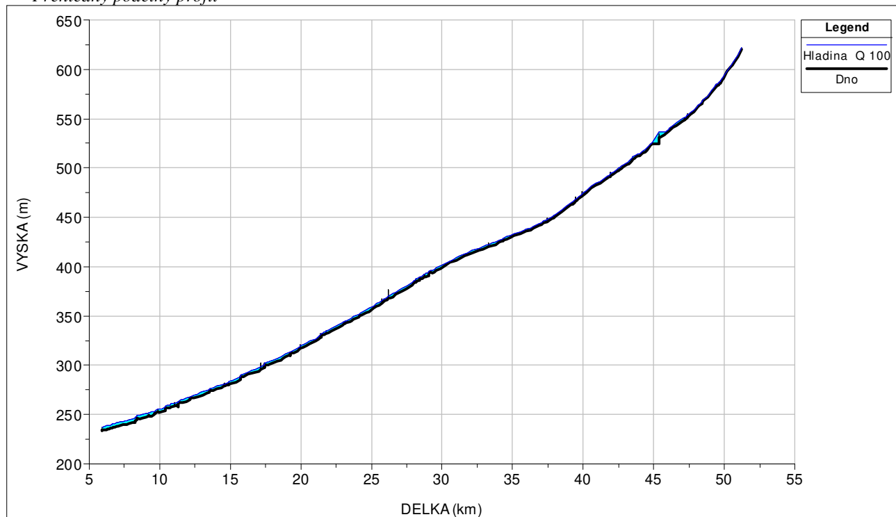
Přehledný podélný profil
